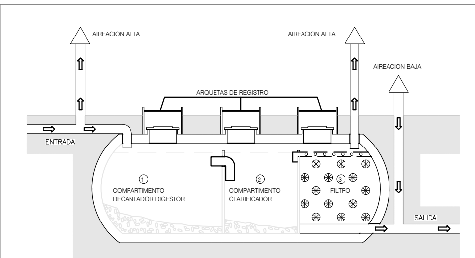
SECCION TRANSVERSAL FOSA SÉPTICA+FILTRO BIOLÓGICO
