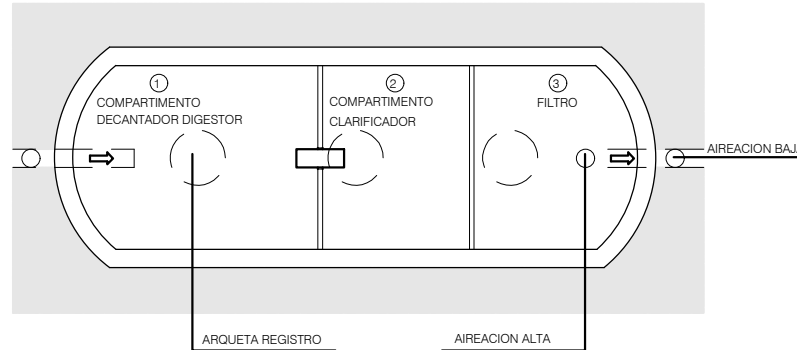
PLANTA FOSA SÉPTICA+FILTRO BIOLÓGICO CAPACIDAD: 3.400lit. (10 pers. ver tabla)
